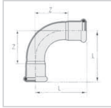
ELBOW 90° f/f
