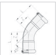
ELBOW 45° f/f
